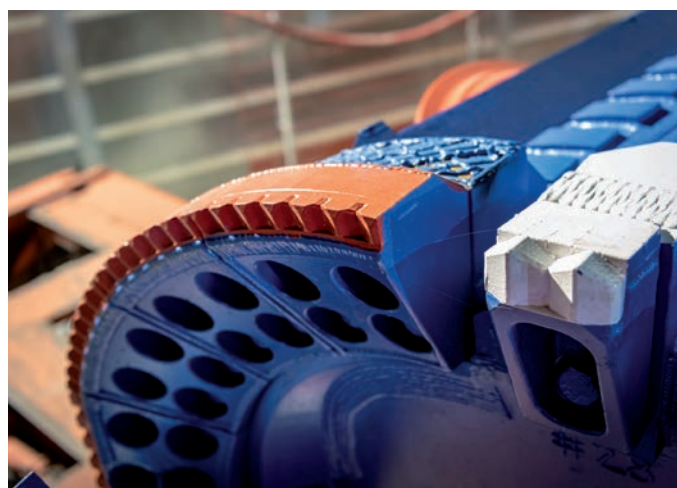
La roue de coupe est composée de nombreux rabots, molettes, couteaux et racleurs, qui attaqueront les différents matériaux rencontrés sur le trajet souterrain du tunnelier.
