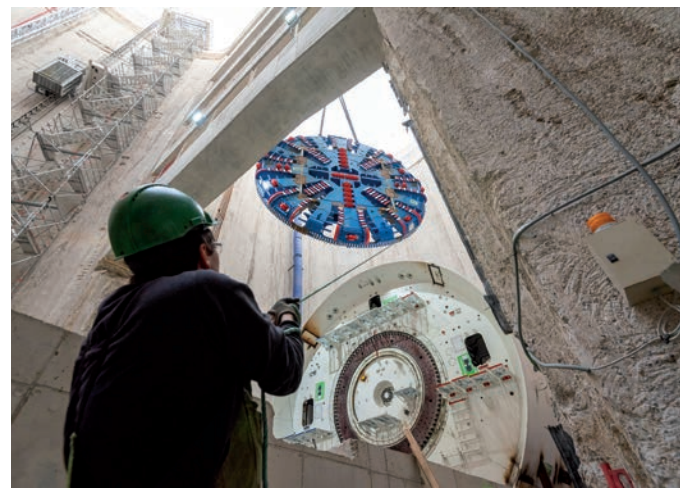
Derrière elle, des voussoirs seront posés au fur et à mesure pour consolider immédiatement les parois du tunnel. Ces arceaux métalliques seront acheminés en parallèle de la remontée des déblais.
